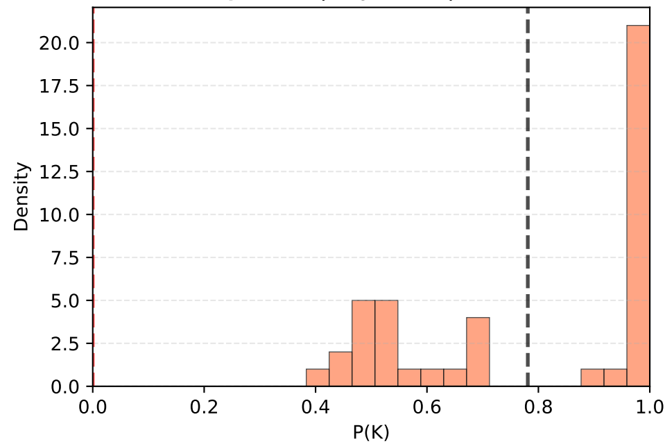
J(K vs R) - ILSP \mu : 0.781 | Obj: 0.000 | n=43
