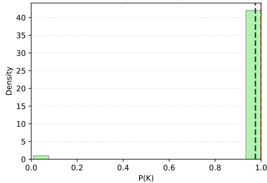
J(K vs R) - LSP \mu : 0.975 | Obj: 1.000 | n=43
